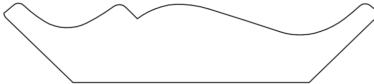
KL 19330 .844 x 4.000 2.875 2.813
