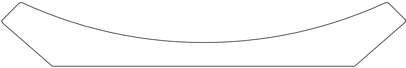
KL 7325 1.063 x 6.750 4.813 4.813
