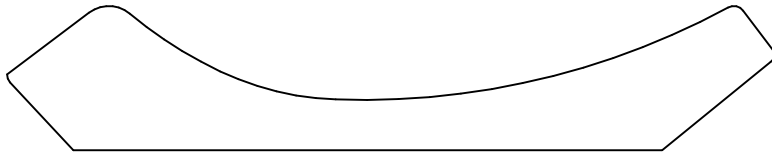
KL 14317 .750 x 4.000 3.125 2.563
