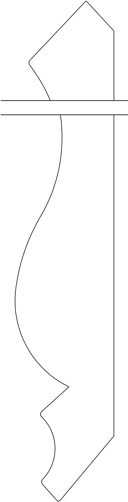
KL 15320 1.750 x 9.188 7.125 5.813
