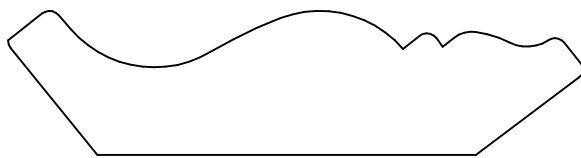
KL 7366 .750 x 3.000 2.313 2.000
