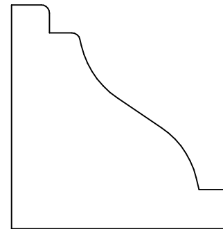
KL 4346 1.687 x 1.625
