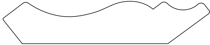
KL 1302 .750 x 3.625 3.000 2.125
