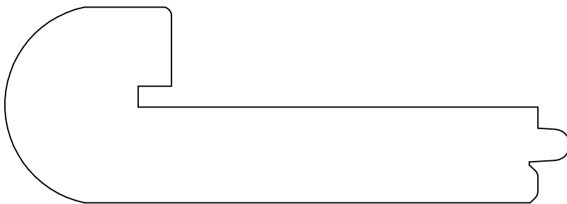
KL 4641 1.469 x 4.240
