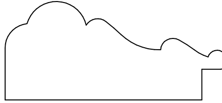
KL 669 1.000 x 2.250
