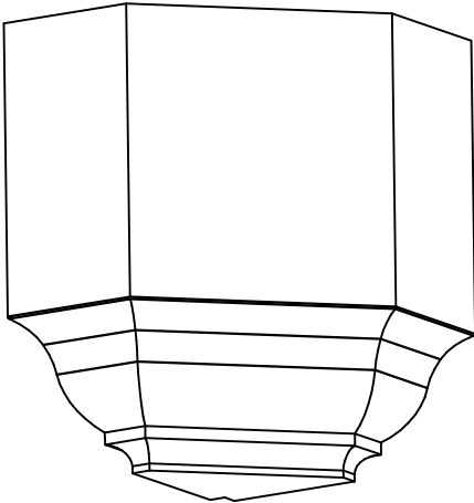
KL CB-3-OC 3.187 x 3.187 x 4.312
