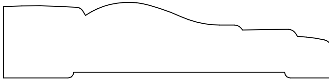
KL 1186 .812 x 3.500
