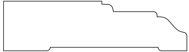
KL 1154 .875 x 3.187
