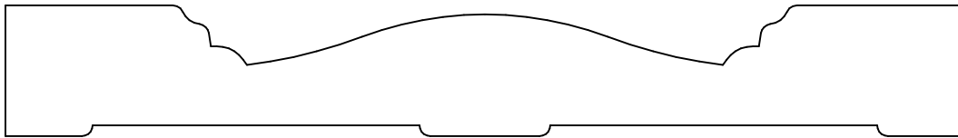
KL 1169 .750 x 5.500
