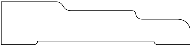
KL 19136 .750 x 3.250
