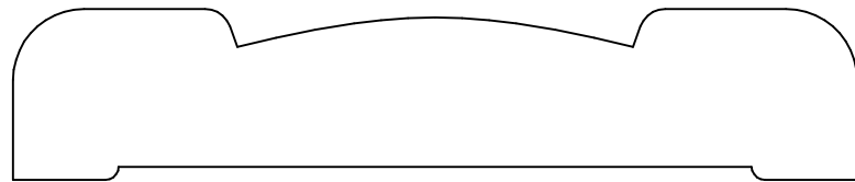
KL 6105 .812 x 4.000
