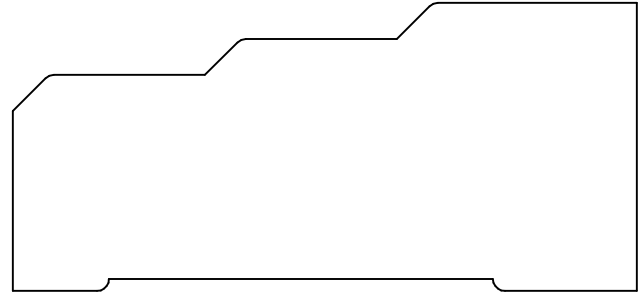
KL 1120 1.500 x 3.250
