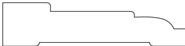
KL 19162 .750 x 3.125
