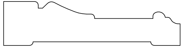
KL 17127 .750 x 3.000
