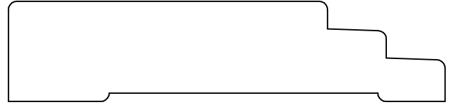
KL 4110 .750 x 3.250
