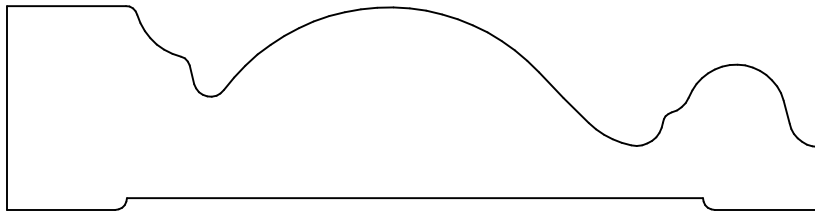
KL 19101 1.063 x 4.250
