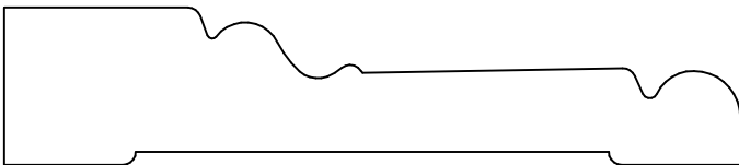
KL 19103 .750 x 3.500
