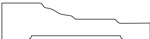
KL 7187 .625 x 2.500
