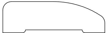
KL 9149 .687 x 2.250
