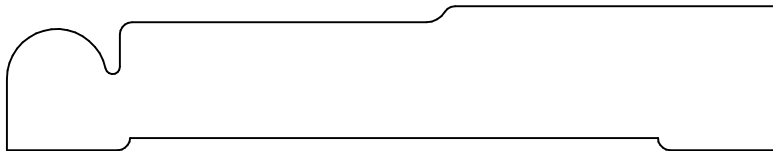
KL 17191 .750 x 4.031
