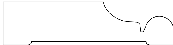
KL 7188 .750 x 3.000
