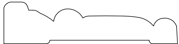
KL 156 .750 x 3.062
