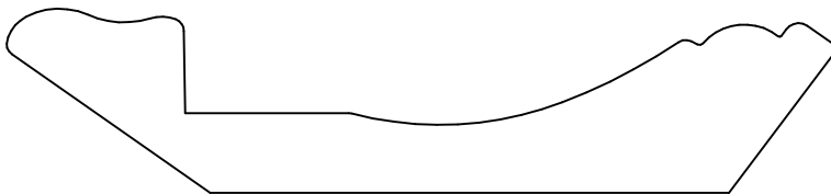
KL 17311A .875 x 3.937 3.250 2.313
