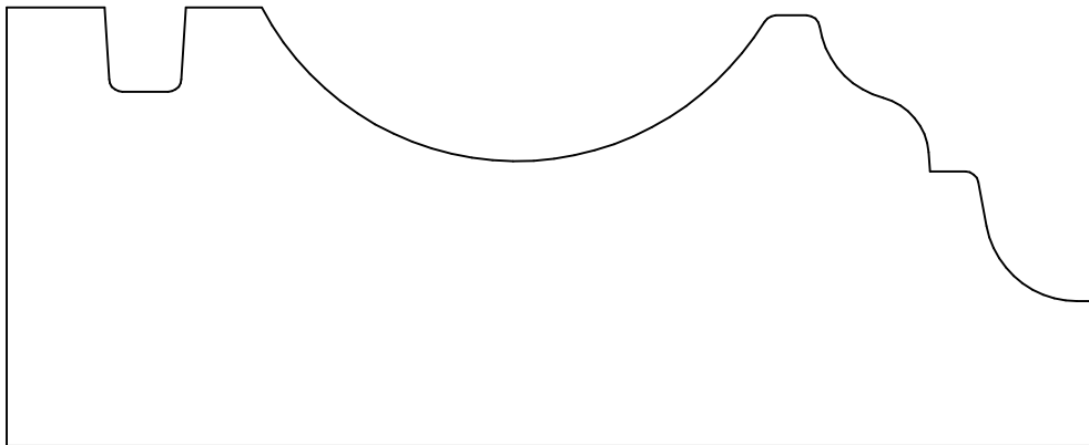
KL 7310-A 2.063 x 5.125
