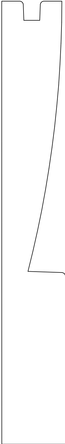
KL 9319-B 1.125 x 7.830
